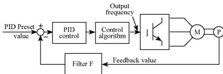
Диаграмма ПИД-регулирования
